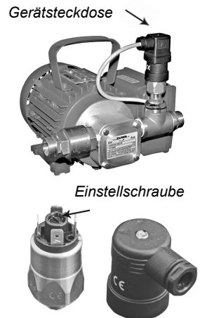
Druckschalter und Gerätesteckdose
