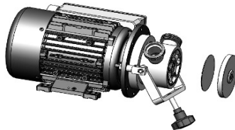
Impellerpumpe NIROSTAR 2000-Cplus
